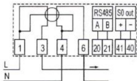
Рис. 1. Схема підключення лічильника
