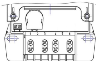
Рисунок 3.2 – Нумерация контактов счетчика в корпусах S7
