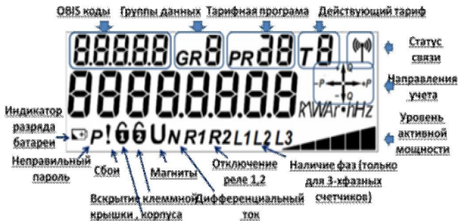
Рисунок 3.3 - Информация, выводимая на дисплей счетчика.
