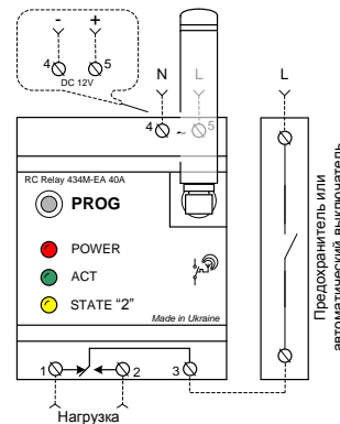
Рис. 1. Схема подключения реле при In ≤ 40А.
