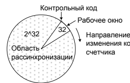
Рис. 6. Диаграмма синхронизации счетчика брелока с контрольным кодом.
