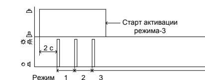
Рис. 4. Диаграмма сигналов реле при выборе режима-3.
