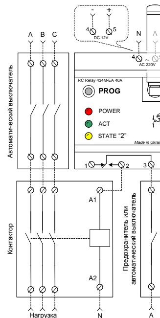
Рис. 2. Схема подключения реле при In > 40А.
